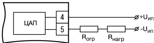
Рисунок 5.4 – Схема подключения ВУ типа И
